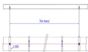
Schéma supportage avec CABS, TIFI
